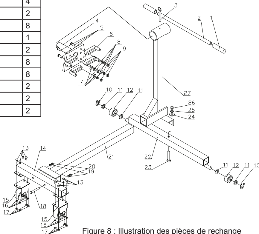
Figure 8 : Illustration des pièces de rechange du modèle 30750
