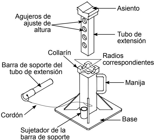
Figure 2 : Componentes del modelo 32225B
