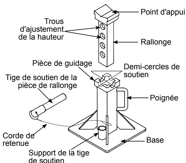
Figure 2 : Composants du Modèle 32225B
