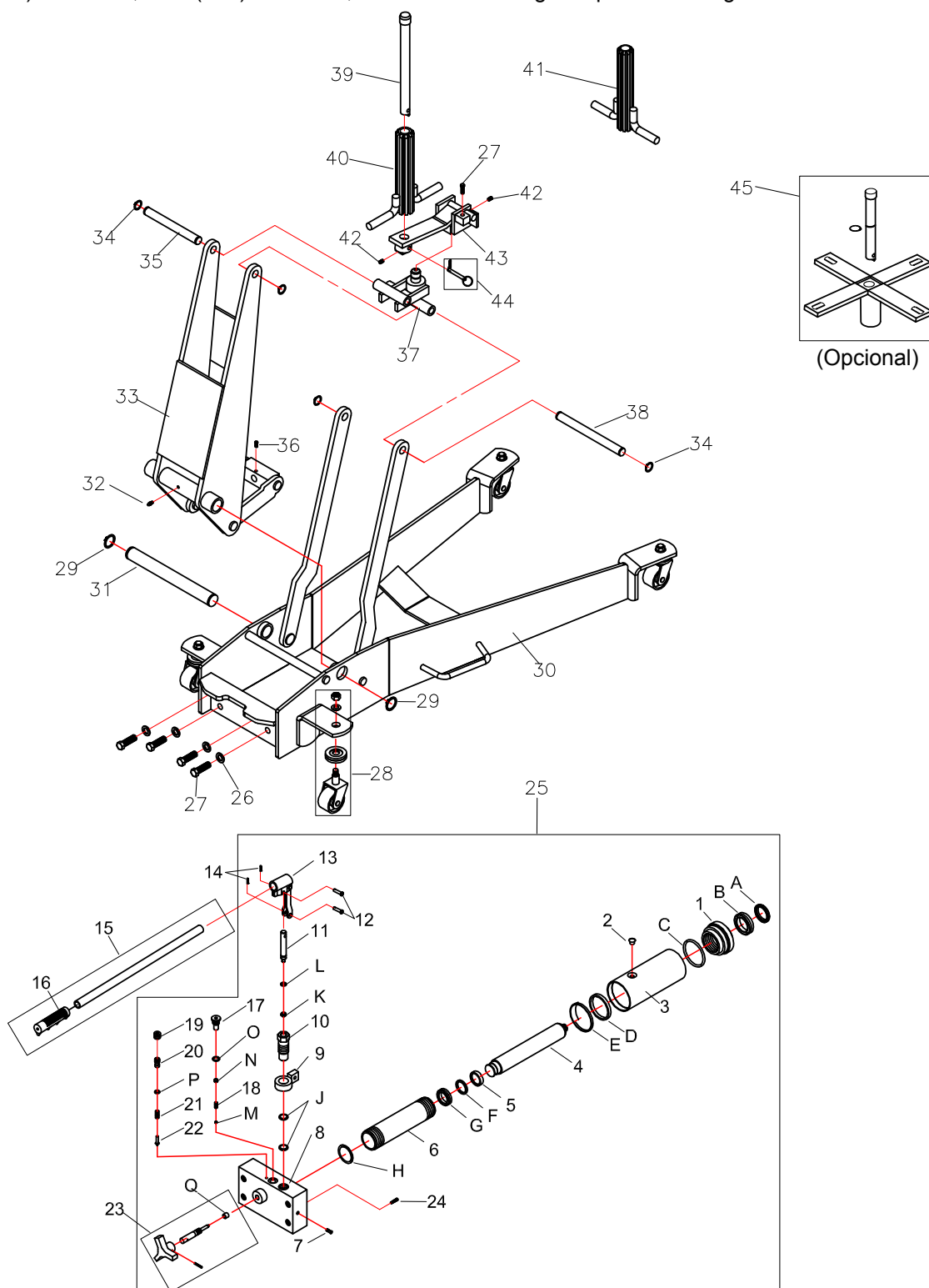
Figura 5: ilustración de piezas de repuesto para el modelo 40500
