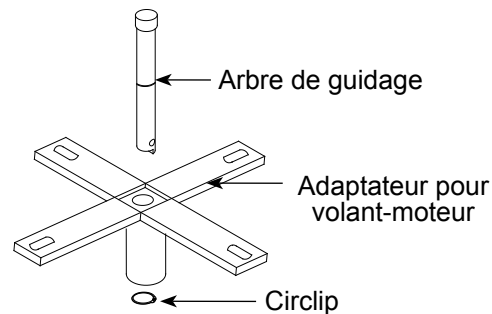
Figure 3 - Composants de l'adaptateur pour volant-moteur
