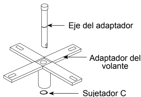
Figura 3: componentes del conjunto del adaptador de volante
