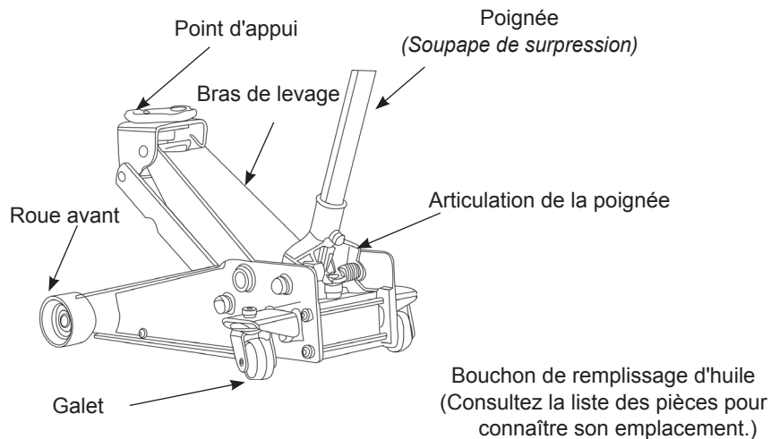
Figure 1 : Pièces d'un cric type
